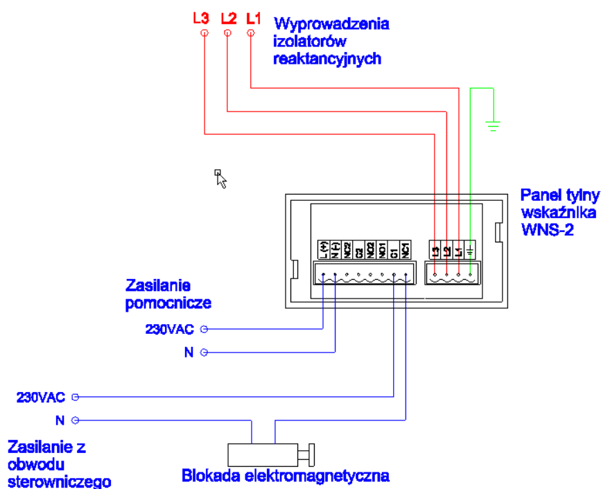
Rys.2. Przykład oprzewodowania wskaźnika napięcia z blokadą łączeniową.
