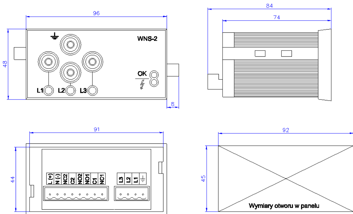
Rys.3. Szkic wymiarowy wskaźnika
